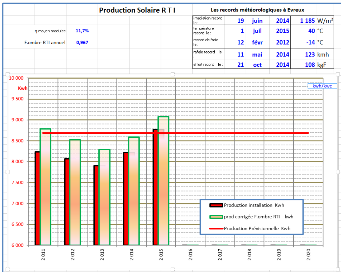
La courbe de production annuelle depuis la mise en service des trackers chez RTI
